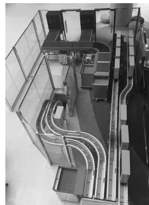
System kolejnic pro automatické pojízdné boxy zajišťuje rychlou distribuci knih uživatelům po knihovně
