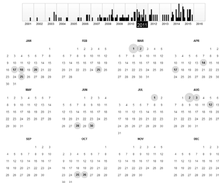
Obr. 4: Aplikace OpenWayback
