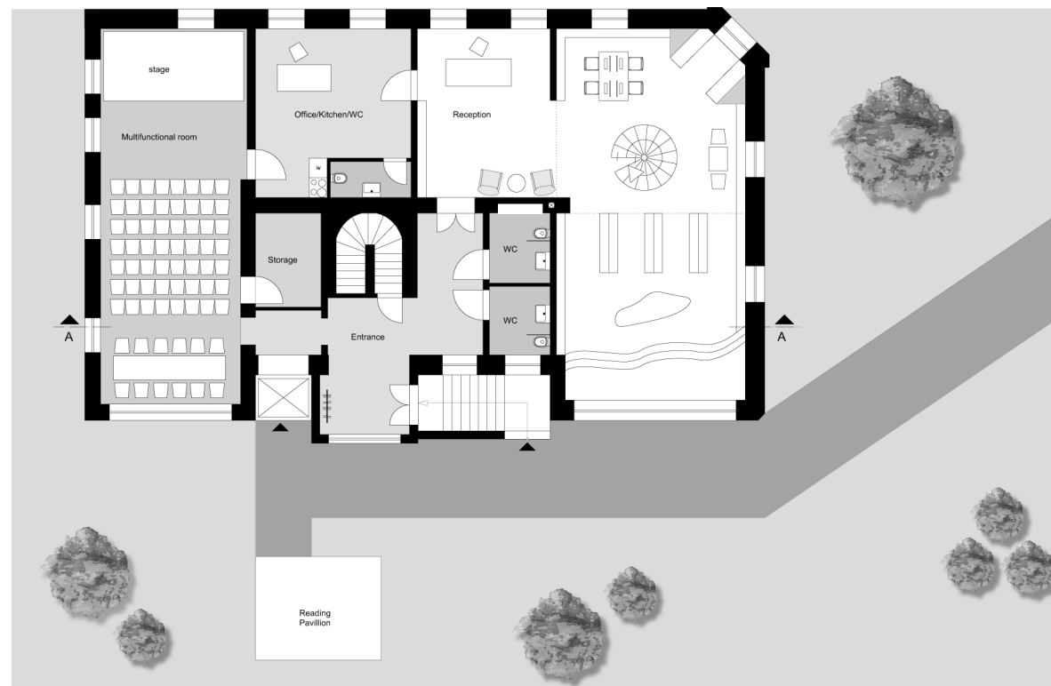
Studie dispozičního řešení v Místní knihovně ve Vranově nad Dyjí Autoři: Žiga Kodelič, Corinna Heller, Anna-Katharina Mathieu, ing. arch. Jan Kratochvíl
