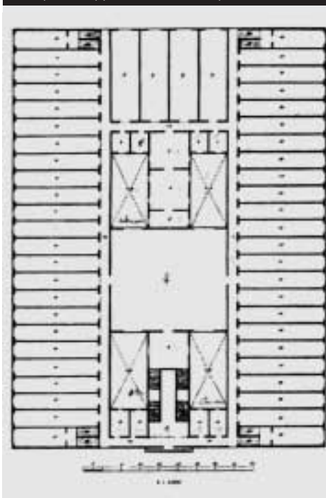
Půdorys knihovny podle návrhu della Santy
